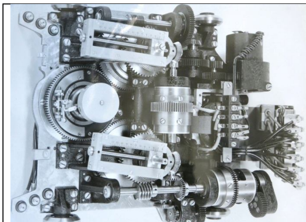
Der Entfernungsmesswagen von nahe, alle vier Räder sind sichtbar. Es ist fast Vorhalt null eingestellt. Zwischen den Flugrichtungsarmen ist die Messrolle, die weiter unten den Flugweg abspult; sichtbar sind ihre feinen Elektrokontakte, welche den Motor steuern zur Einstellung der Flugrichtungsarme. Die beiden Arme müssen exakt parallel sein, da ist etwas noch nicht richtig justiert. Ungarisches Fotopapier Gamma-Juhasz, spiegelt leicht. FF-Museum Dübendorf.
