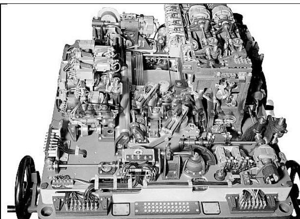
Der Entfernungswagen (Bildmitte), eingebaut in ein Kommandogerät mit Kurven-Berechnung (hier sind die beiden Flugrichtungsarme schräg versetzt). Hinter dem Wagen der nötige Platz zur Verschiebung, darunter die feste Platte, auf der die Messrolle läuft. Links vier Schienen für Elektrokontakte (Messrolle), es hat lange Zahnwalzen zur Übertragung der Daten auf den fahrenden Wagen. Hasler-Bild, Museum f. Kommunikation
